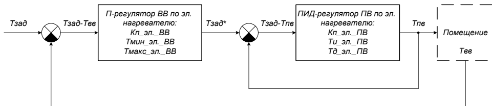
Рис.4.9. Структурная схема регулятора ВВ по эл. нагревателю
