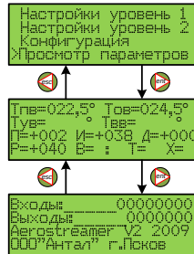
Рис.4.11. Меню «Просмотр параметров»
