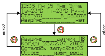
Рис.4.12. Меню «Просмотр ошибки»
