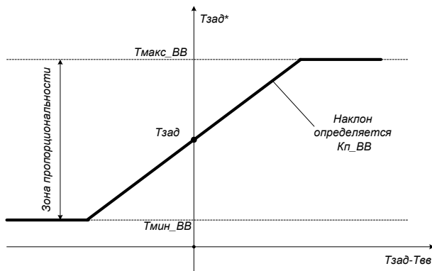
Рис.4.10. К пояснению работы регулятора ВВ
