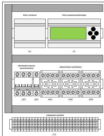
Рис. 2.2. Эскизный чертеж ящика управления
