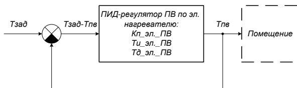
Рис.4.7. Структурная схема регулятора ПВ по эл. нагревателю
