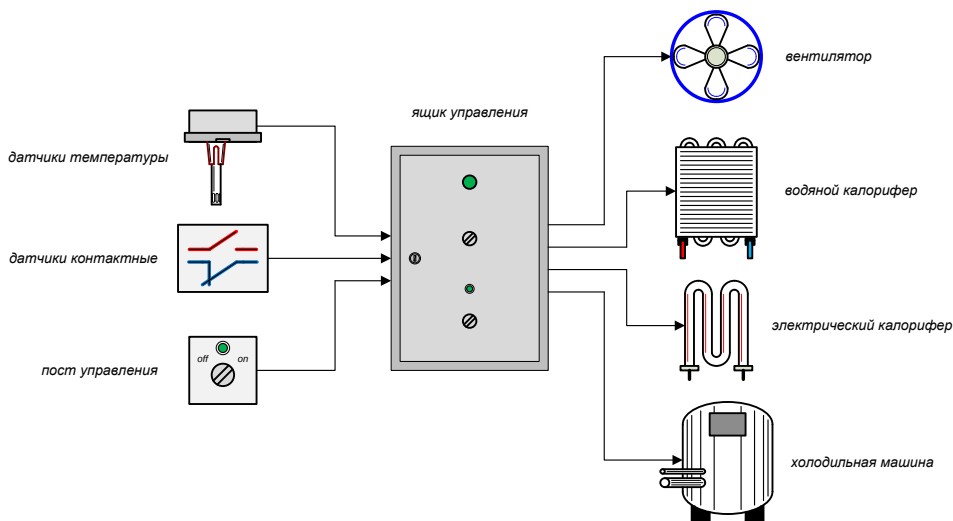
Рис. 2.1. Упрощенная структура системы
