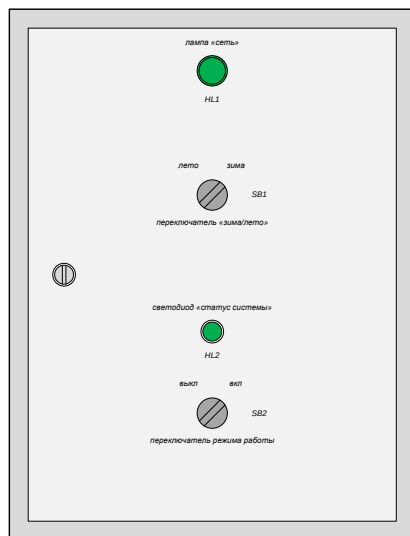
Рис. 2.3. Эскизный чертеж передней панели ящика управления
