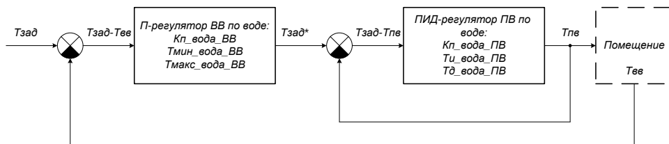
Рис.4.8. Структурная схема регулятора ВВ по воде
