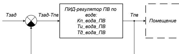
Рис.4.6. Структурная схема регулятора ПВ по воде
