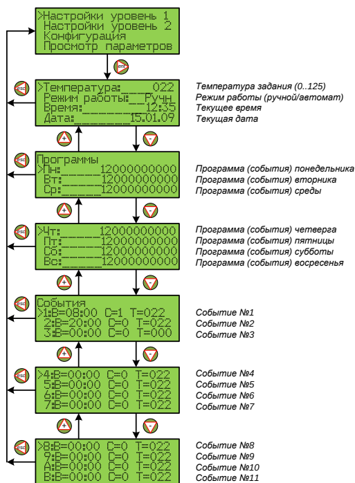
Рис.4.2. Группа меню «Настройки уровень 1»
