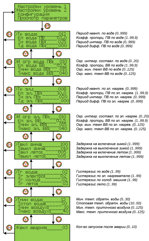
Рис.4.3. Группа меню «Настройки уровень 2»
