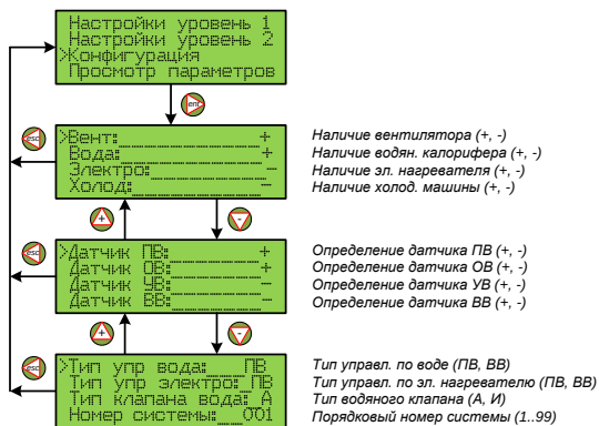
Рис.4.4. Группа меню «Конфигурация»
