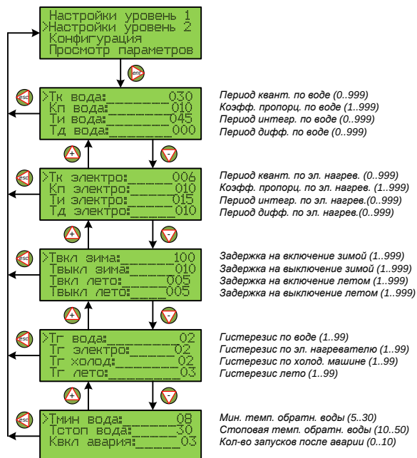
Рис.4.3. Группа меню «Настройки уровень 2»
