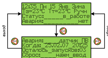
Рис.4.7. Меню «Просмотр ошибки»
