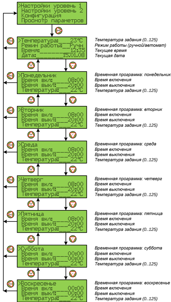
Рис.4.2. Группа меню «Настройки уровень 1»
