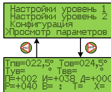
Рис.4.6. Меню «Просмотр параметров»
