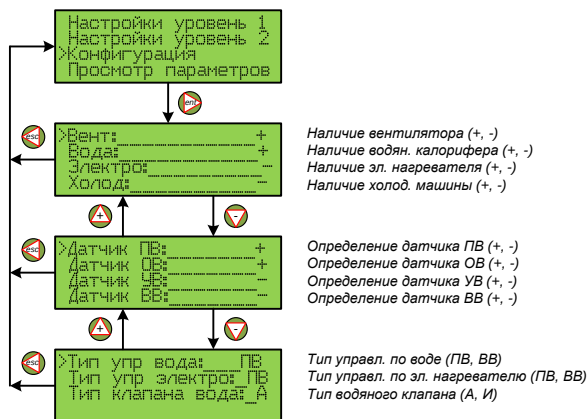
Рис.4.4. Группа меню «Конфигурация»
